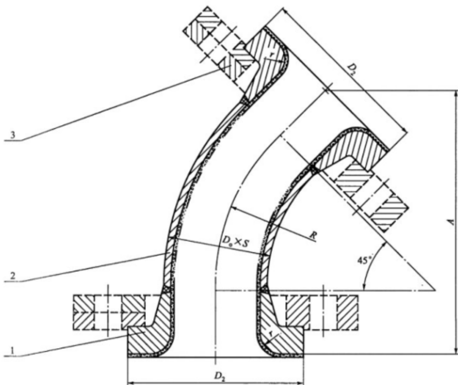
图 1 搪玻璃 45°弯头结构型式图
